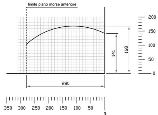
Diagramma di taglio troncatrice Retta con lama Ø 500mm (tolleranza ±3mm)
